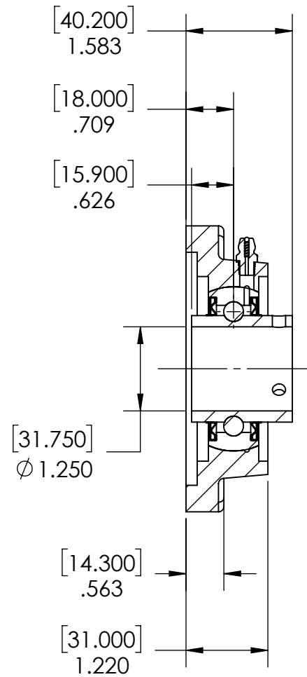
SECTION A-A
